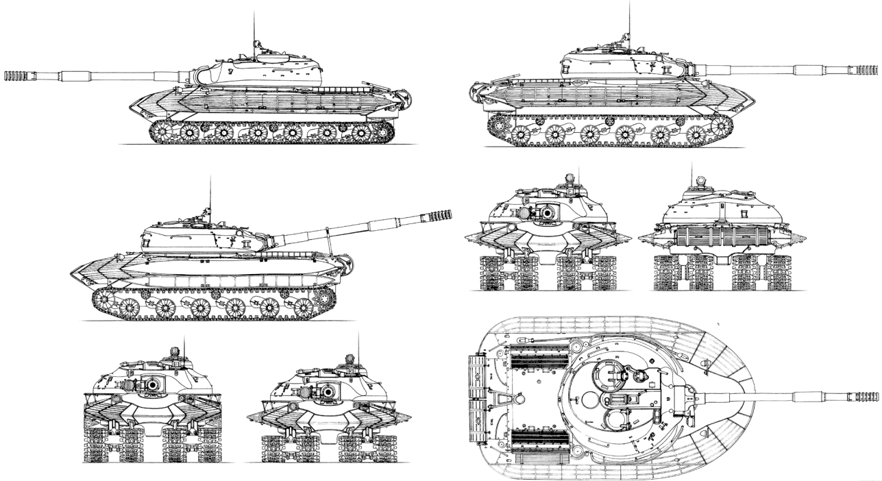
«Объект 279». Развёрнутые проекции.
